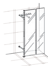
Alba 2 mit Albatros Seitenwand 2 B 85 H 204 T 22
